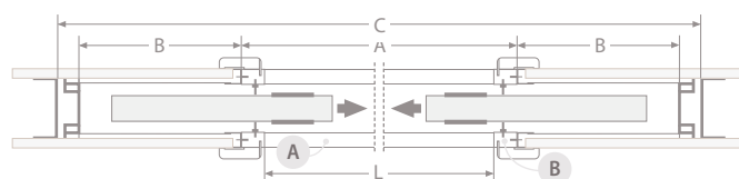
DVOUKŘÍDLÉ DVEŘE (mm)
