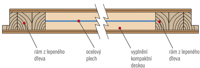
PRÁH Z NEREZOVÉHO PLECHU
