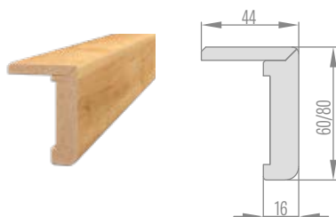
STANDARDNÍ ÚHELNÍK K NASTAVITELNÉ ZÁRUBNĚ
