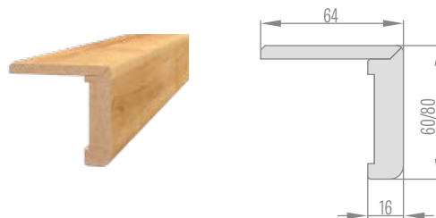
ÚHELNÍK S PRODLOUŽENÝM JAZÝČKEM DO NASTAVITELNÉ ZÁRUBNĚ
